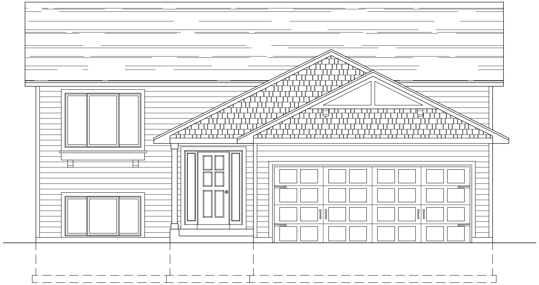
FRONT ELEVATION N.T.S.
